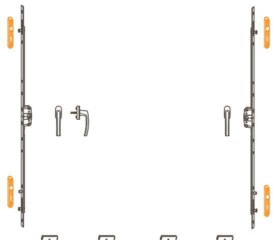
Herraje 2 hojas para corredera lineal
