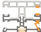
Guía persiana cajón con mosquitera
