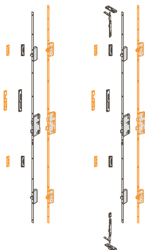
Herrajes para puerta de calle
