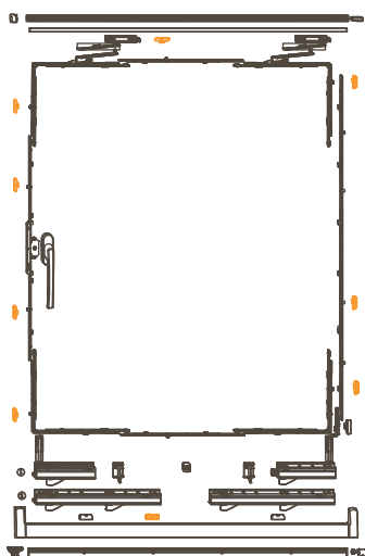
Herraje Oscilobatiente Seguridad básica 1 hoja
