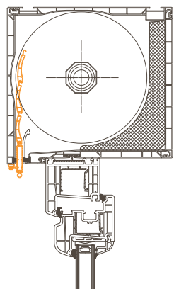
Detalle sección cajón persiana
