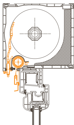
Detalle sección cajón persiana con mosquitera
